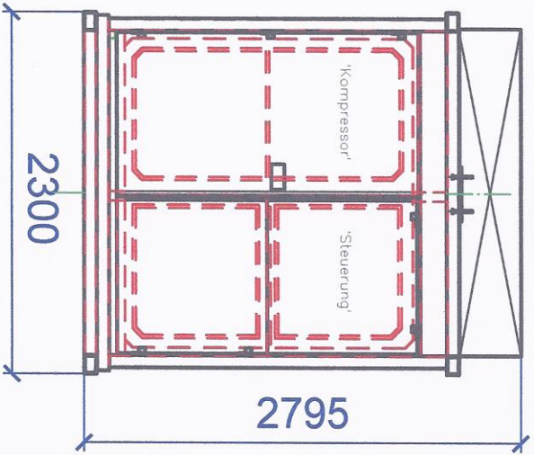
Ansicht Schaltschrank- Seite
