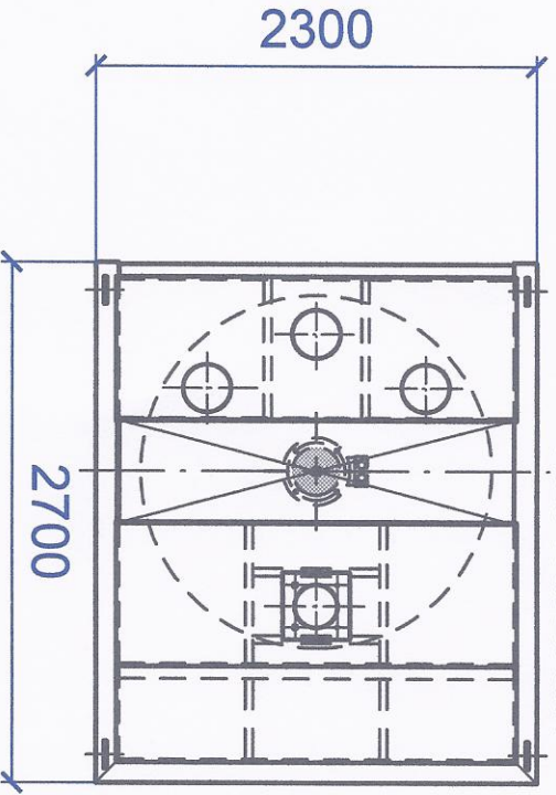
Draufsich Dach, ohne Wassertank
