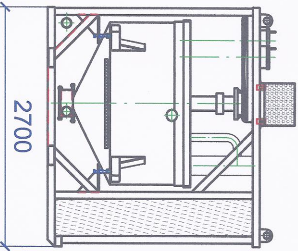
Draufsich Dach, ohne Wassertank
